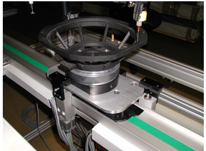
Durch die Indexierung des WT an der Klebestation, ist eine Positionierung von 0,1 mm möglich
