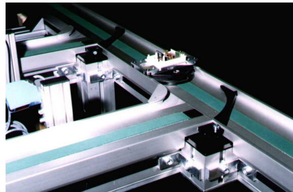
WT - oval zwischen automatisierter und manueller Weiche
