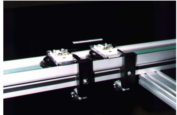
WT - oval an handbetätigtem Doppelstopper zur Vereinzelung am Arbeitsplatz
