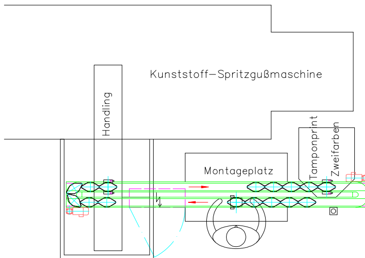
WT- oval an Stopper mit Indexierung der Handling - Station mit Rückstau über die 180°-Kurve
