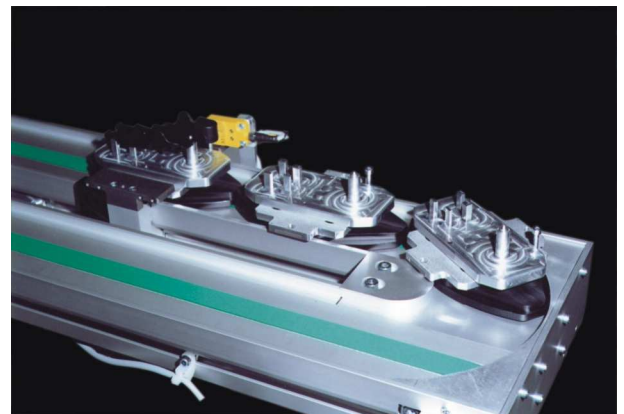
WT- oval an Stopper mit Indexierung der Handling - Station mit Rückstau über die 180°-Kurve
