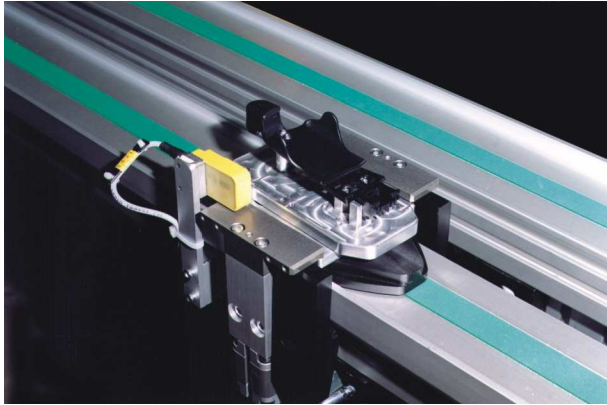
WT- oval an Stopper mit Indexierung der Zweifarbenn - Tamponprint Station
